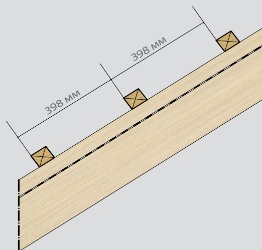
ШАГ ОБРЕШЕТКИ
