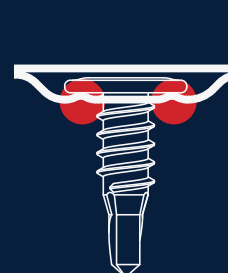
Специальные продольные волнообразные ребра жесткости под шляпку самореза
