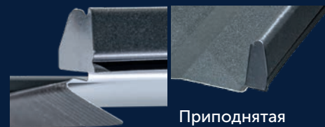
Скрытый элемент замка (панель)
