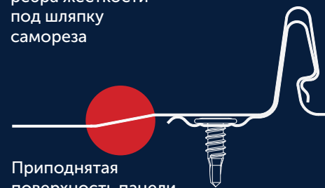
Профилированная кромка верхнего замка
